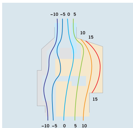
Die Isotherme verlaufen bei den Holz-Metall-Fenstern in einem Bereich, der eine ideale Wärmedämmung garantiert
